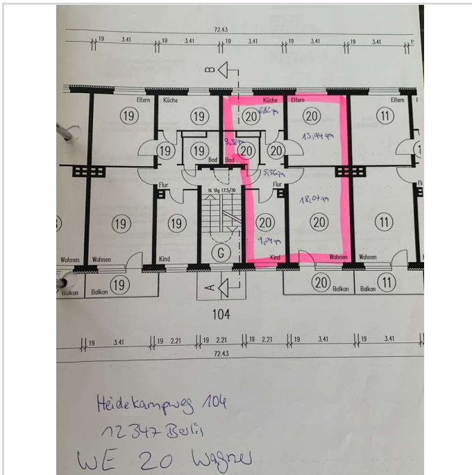
Grundriss Heidekampweg 104
